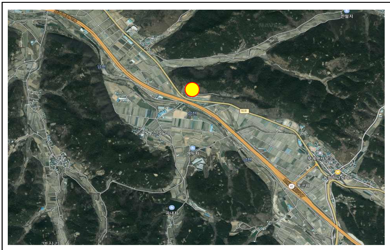
【그림 35.13】 상주절토35 검토대상 비탈면구간
