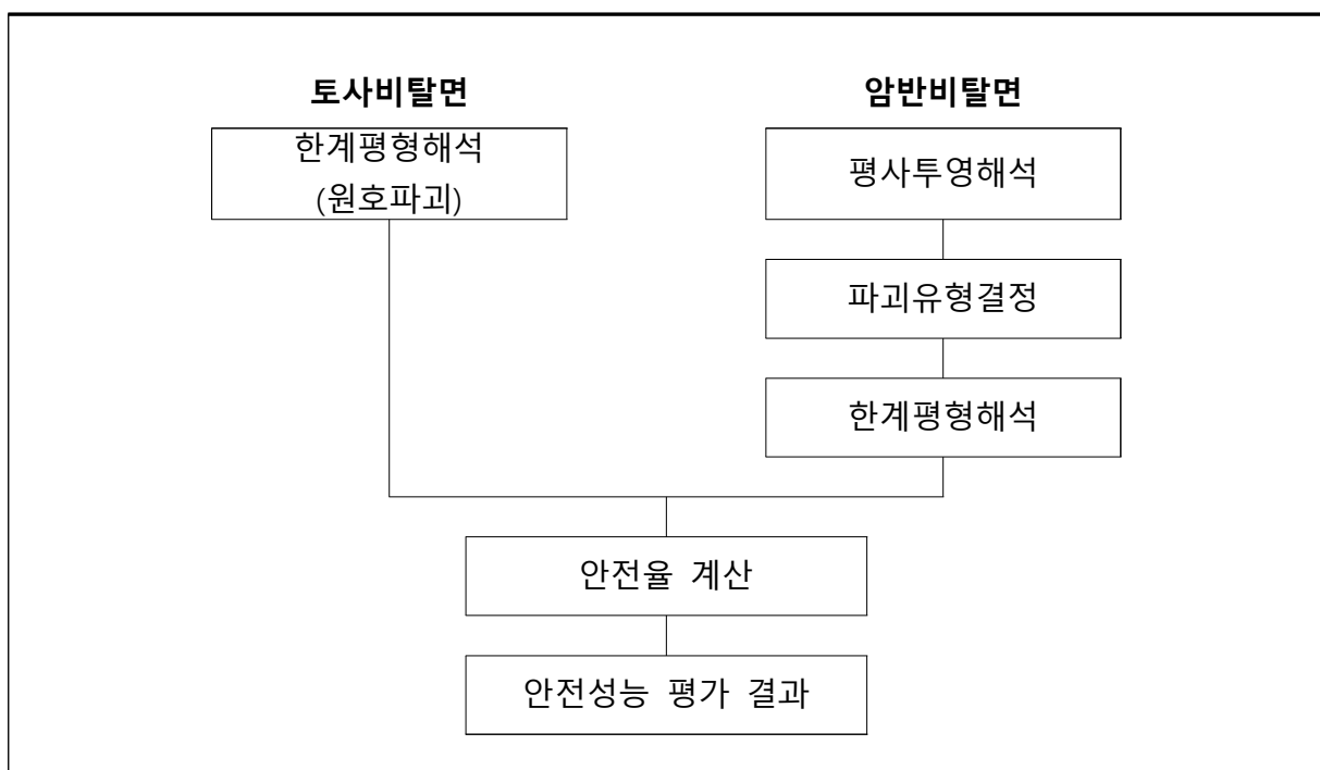
【그림 35.5】 구조안전성능 평가과정
