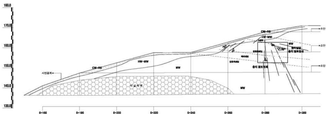
【그림 35.14】 상주절토35 검토대상 비탈면구간
